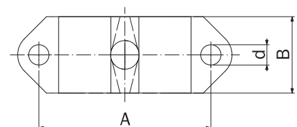
Type GMD-1 und GMD-2 Top view
