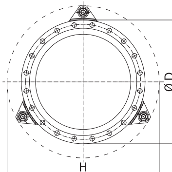
DN 200 - DN 300
