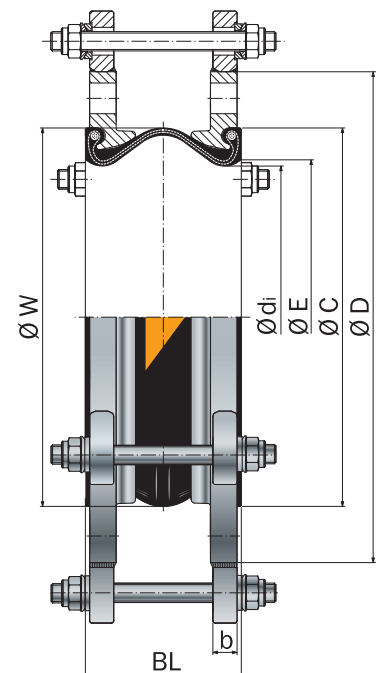
DN 200 - DN 300
